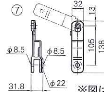
※本体 SCS-13 パフ研磨 ※上カバー SCS-13 電解研磨
