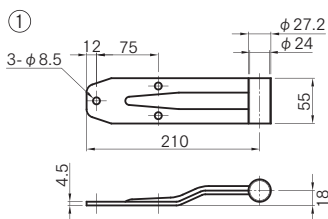
※SS400 3価クロメートメッキ
