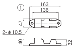
※FCD45 3価クロメートメッキ
