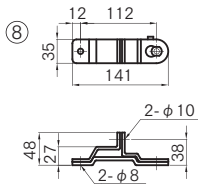
※SUS304 #400研磨
