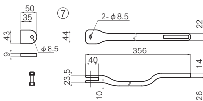
※FCD45 3価クロメートメッキ
