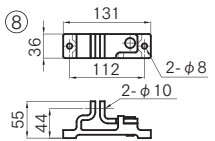
※SCS-13 バフ研磨
