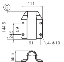
※SPHC 3価クロメートメッキ
