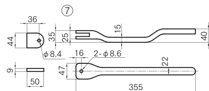
※SCS-13 バフ研磨 SUS M8x35 六角ボルト、SUS M8 Uナット SUS M8用 スプリングワッシャ 付
