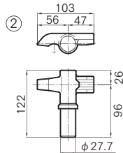
※SCS-13 パフ研磨 ※本図は左用を示す
