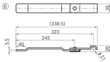
※SS400 3価クロメートメッキ
