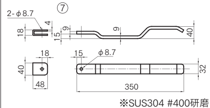
※SUS304 #400研磨
