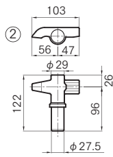
※SCS-13 バフ研磨 ※本図は左用を示す
