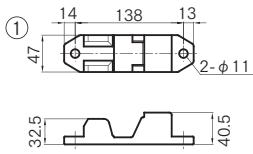
※SCS-13 パフ研磨
