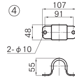
※SPHC 3価クロメートメッキ
