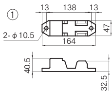
※SCS-13 バフ研磨
