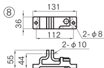
※SCS-13 バフ研磨
