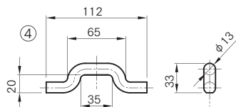
※SS400 3価クロメートメッキ
