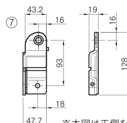
※本図は正側を示す。 ※SS400 3価クロメートメッキ
