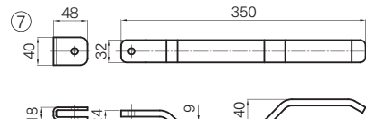
※SUS304 #400研磨 SUS M8x35 六角ボルト、SUS M8 Uナット SUS M8用 スプリングワッシャ 付
