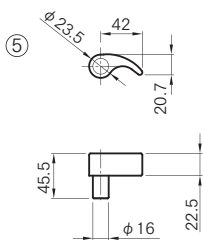
※SS400 3価クロメートメッキ
