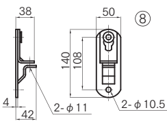
※SUS304 #400研磨
