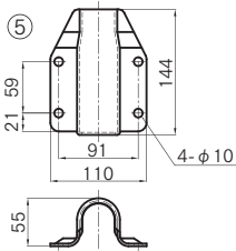
※SUS304 #400研磨
