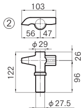
※SCS-13 パフ研磨 ※本図は左用を示す
