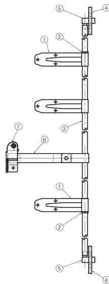
※本組立図は正側を示す
