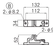
※FCMB32 3価クロメートメッキ
