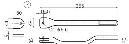
※SCS-13 パフ研磨
