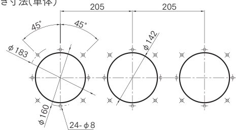
取付切欠き寸法(単体)
