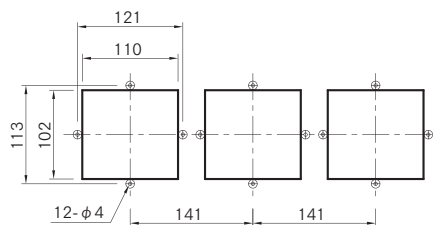
取付切欠き寸法( 単体 )
