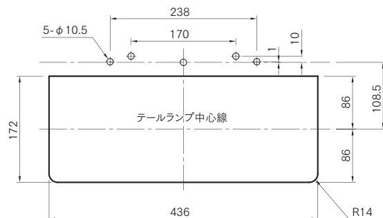
取付切欠き寸法( Assy )
