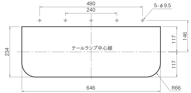
取付切欠き寸法(ASSY)
